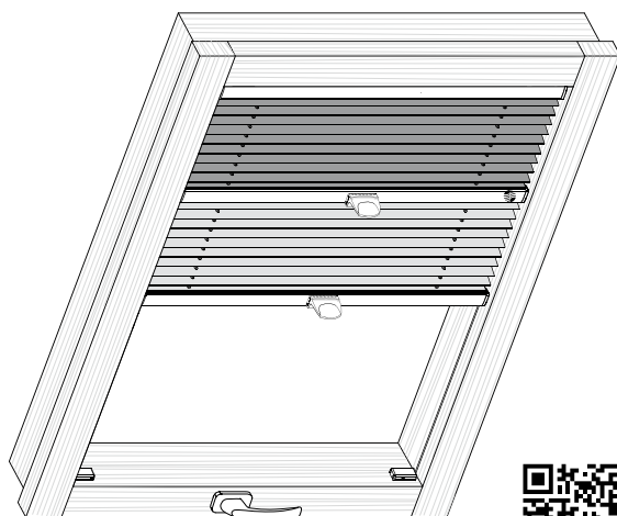
Plissee Typ 2620 mit Spannschuhplättchen-Clip
